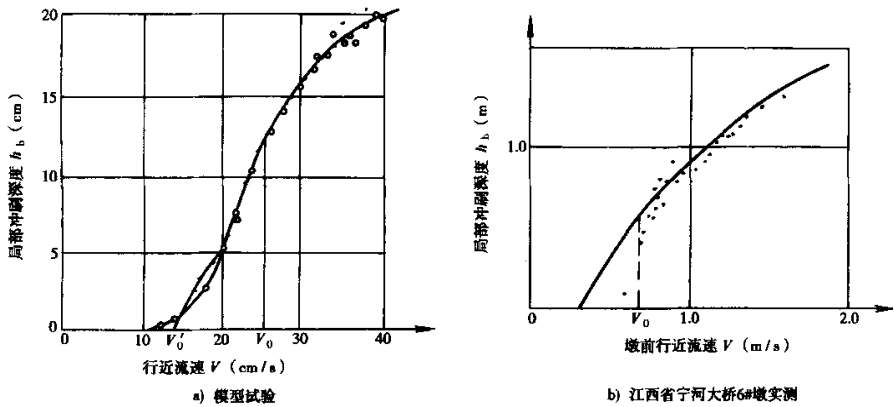
图2 桥墩局部冲刷深度与行近流速的关系
