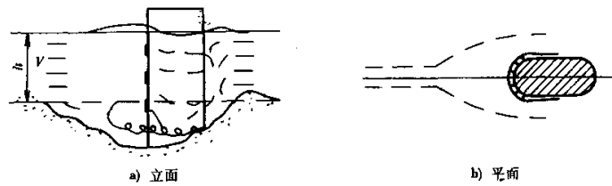
图 1 桥墩局部冲刷示意图
